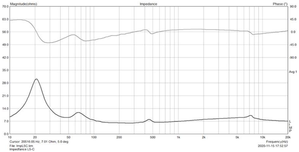
Courbes de phase et d'impédance
